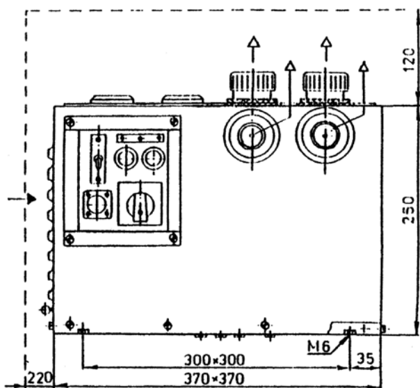
Mobilní filtroventilační komplet FVZ MK 15/24
